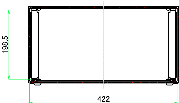
B-B ( 1 : 6.5 )
